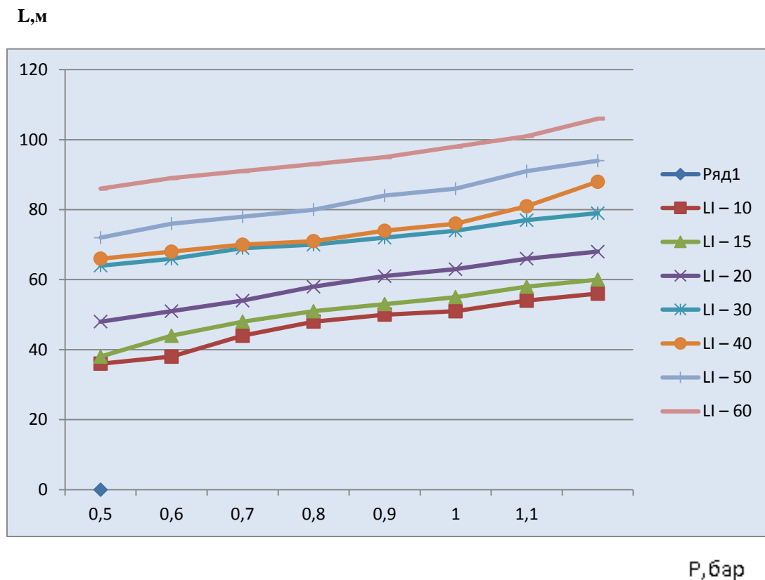
График зависимости дальности струи L,м от давления P,бар
